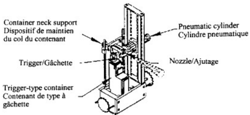
FIGURE 3 Appareil de maintien pour contenant de type à gâchette Vue isométrique
